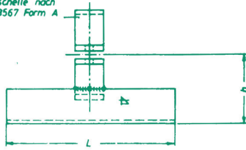
Rohrschelle nach DIN 3567 Form A
